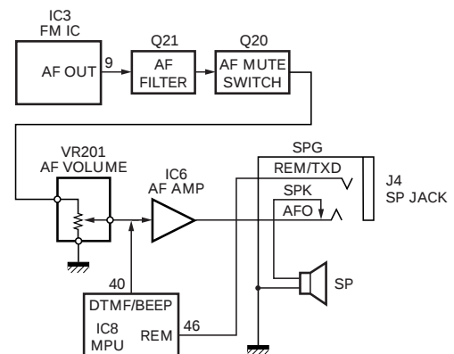
Fig. 4 AF amplifier
